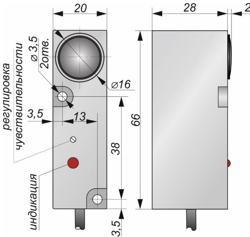
Габаритный чертеж
