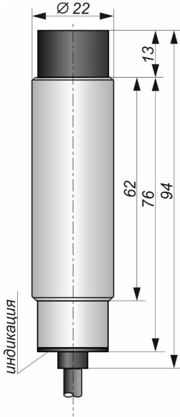
Габаритный чертеж
