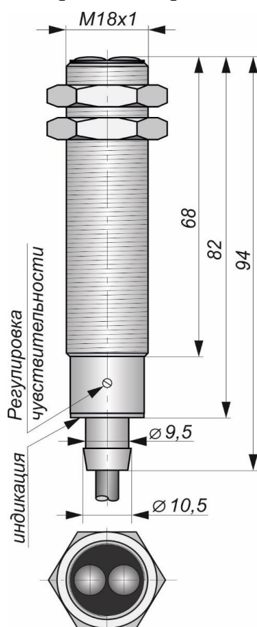
Габаритный чертеж
