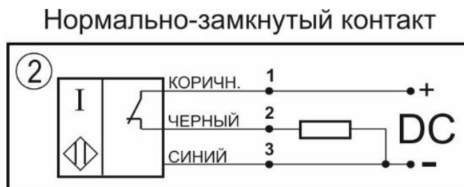
Схема соединения
