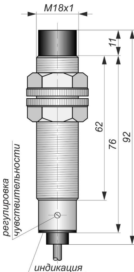
Габаритный чертеж
