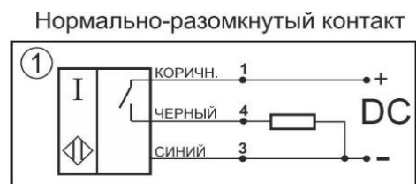
Схема соединения
