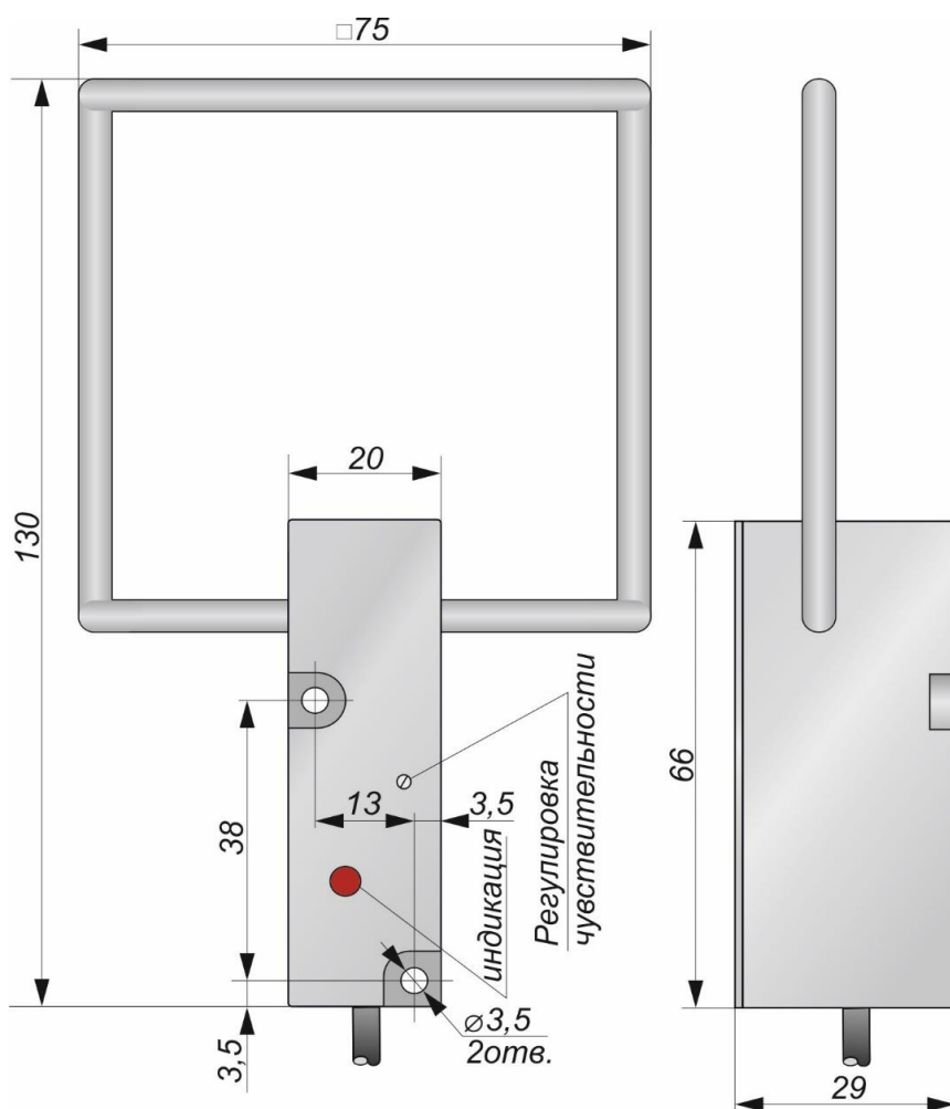
Габаритный чертеж
