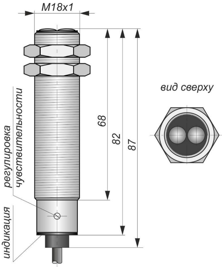
Габаритный чертеж
