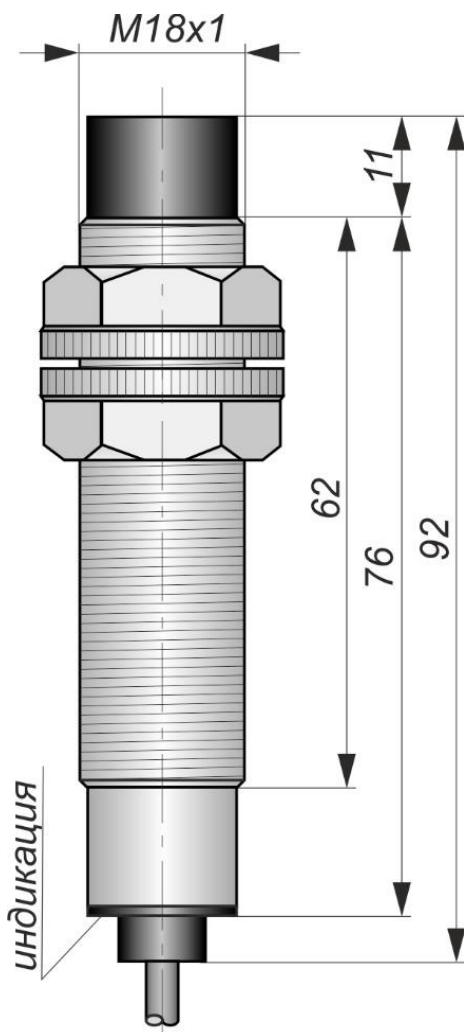
Габаритный чертеж
